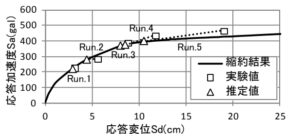
図－5 縮約結果と実験値・推定値の比較
