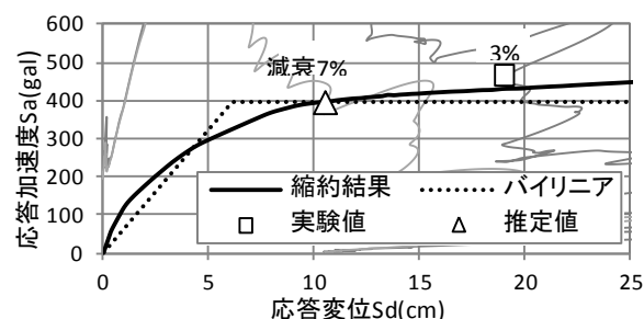
図－6 等価線形化法による応答推定 (Run. 5 の例)
