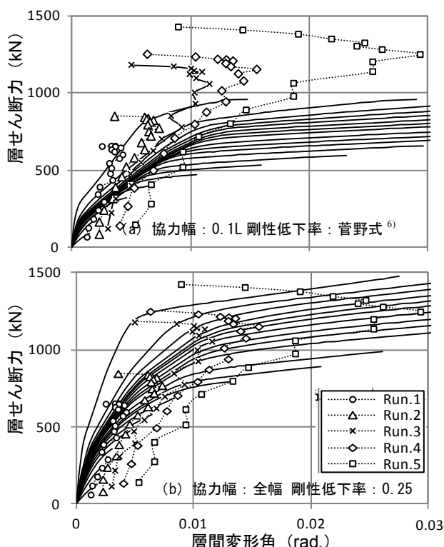
図一4 層せん断力-層間変形角と各 Run の最大応答点
