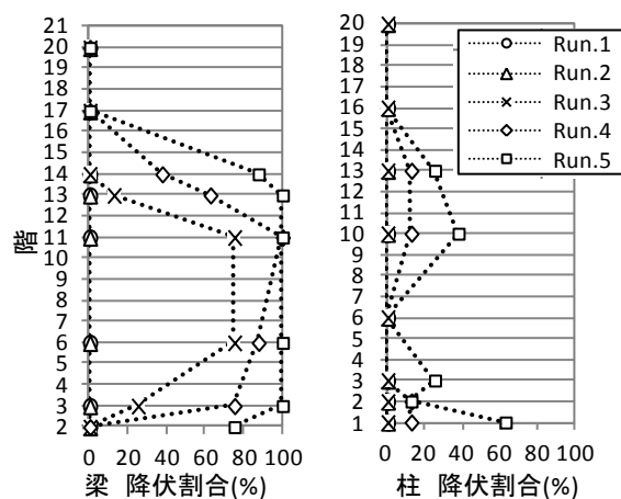
図一3 降伏状況の推移
