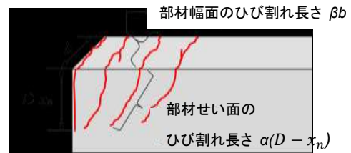
図-14 ひび割れ長さ評価モデルの概要
